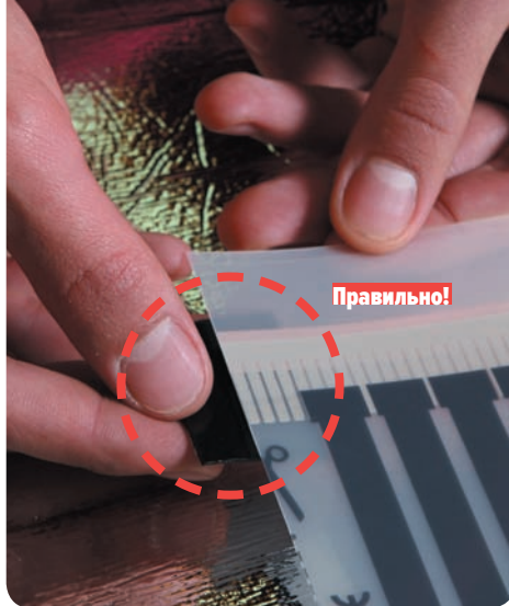
Рис. 12. Пример правильной установки изоляции линии отреза медной шины
