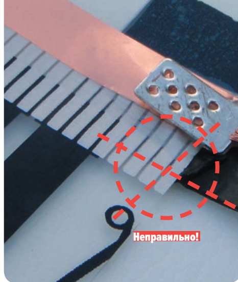
Рис. 18. Пример неправильной установки нижнего листа изоляции контактных зажимов
