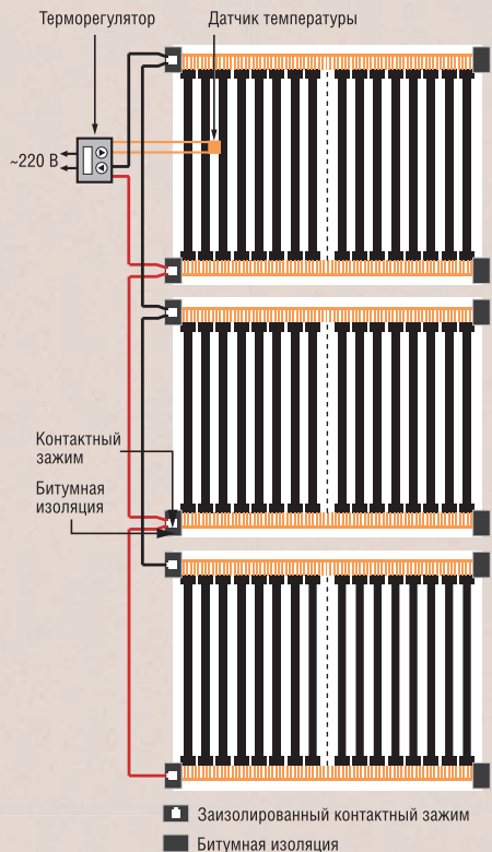
Рис.5. Общая схема подключения термопленки CALEO
