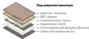
Рис. 29. Схема монтажа теплого пола CALEO под ковролин или линолеум
