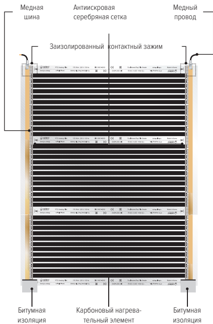
Рис. 3. Общий вид термоматки CALEO, расположение основных ее элементов, контактных зажимов и мест подключения и изоляции
