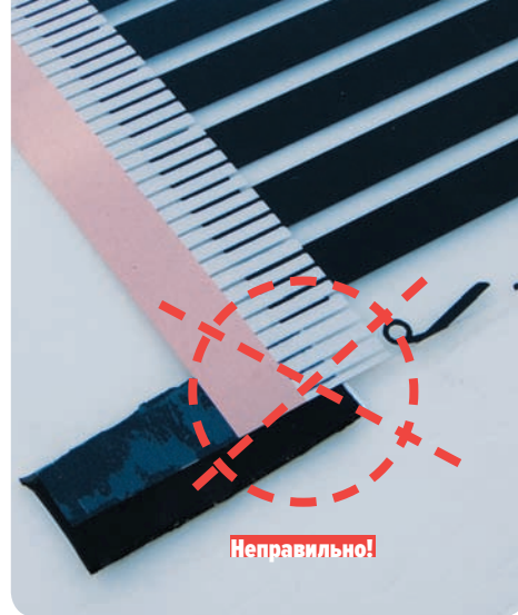
Рис. 13. Пример неправильной установки изоляции линии отреза медной шины
