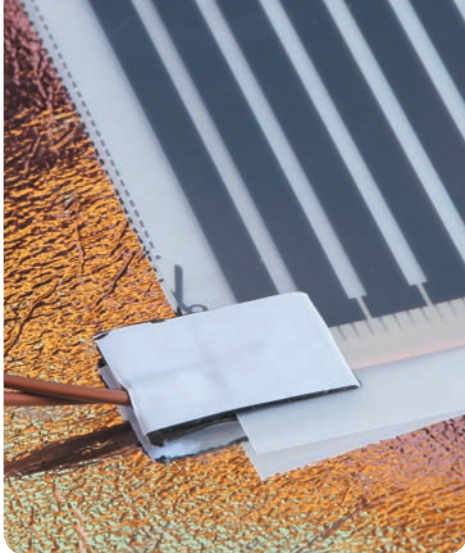
Рис. 20. Вид заизолированного контактного зажима с подключаемыми проводами
