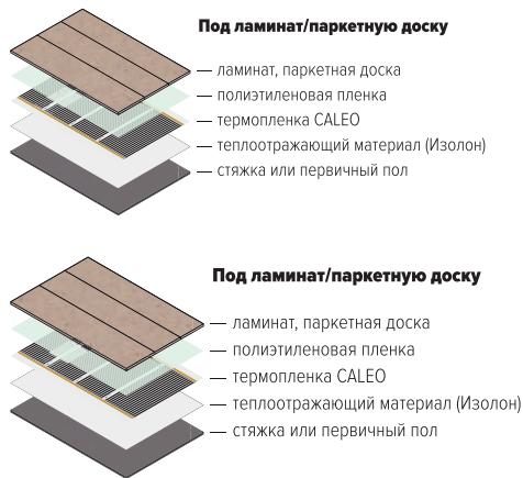
Рис. 4. Схема монтажа теплого пола CALEO под ламинат, ковровин, линолеум
