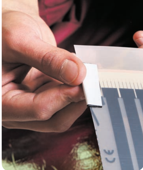
Рис. 14. Окончание процесса изолирования линии отреза медной шины
