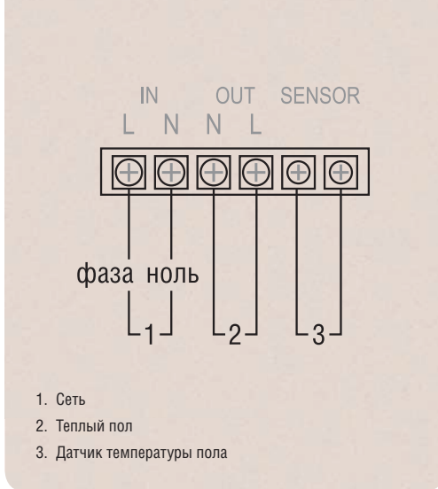
Рис. 21. Пример подключения соединительных проводов к терморегулятору CALEO Model 320
